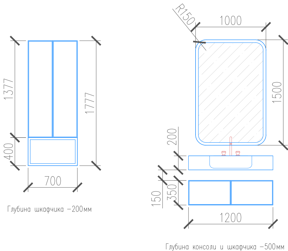
Санузел 1
