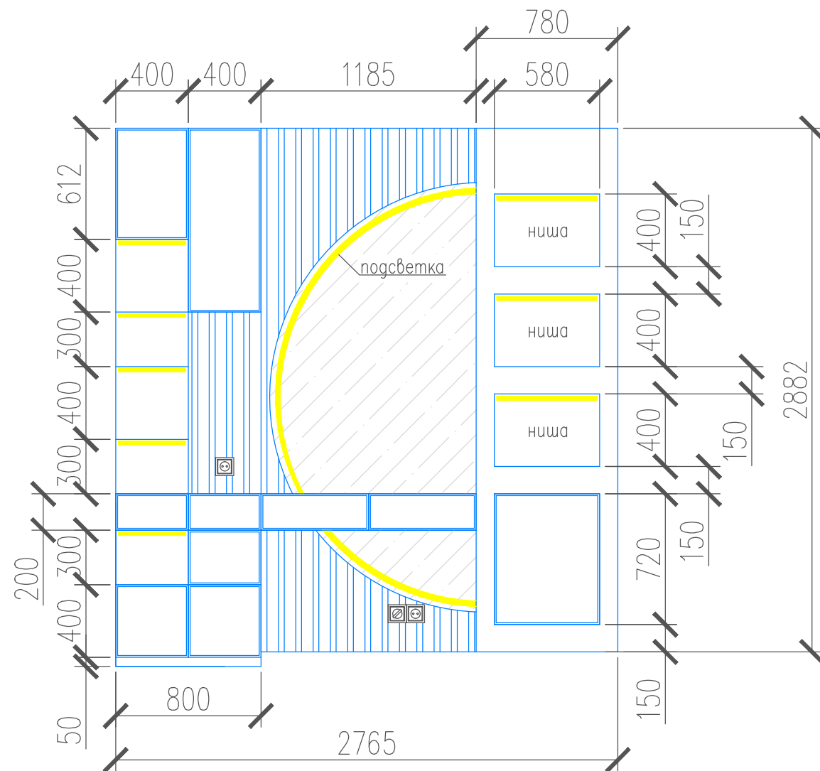
Мебель в прихожей-холле
